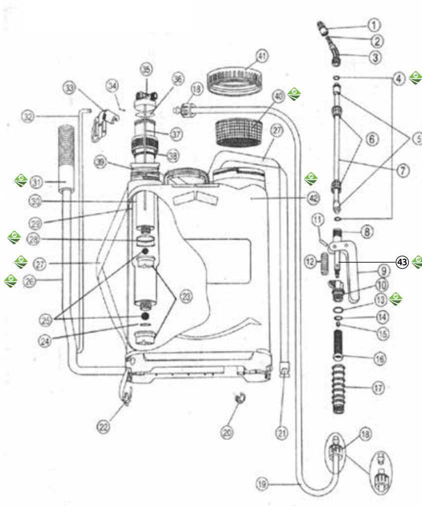
Modelo: 3WBS-20
